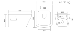
VITO MINI Wall Hung Closet 500x355x350mm 20"x14"x14" 26.00 Kg.
